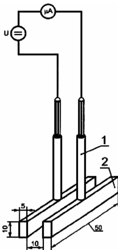
1 - изоляция; 2 - латунные электроды. Предельные отклонения размеров \pm 1 мм.
